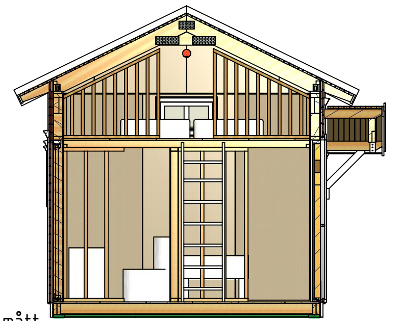
C-C ( 1 : 50 )
