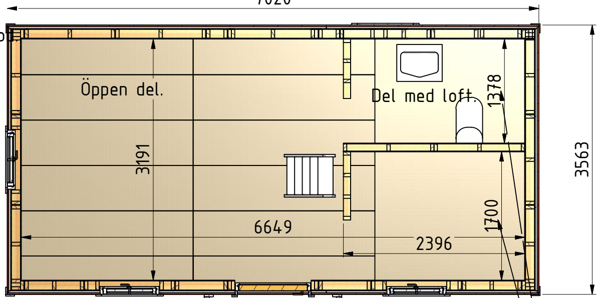
B-B ( 1 : 50 )
